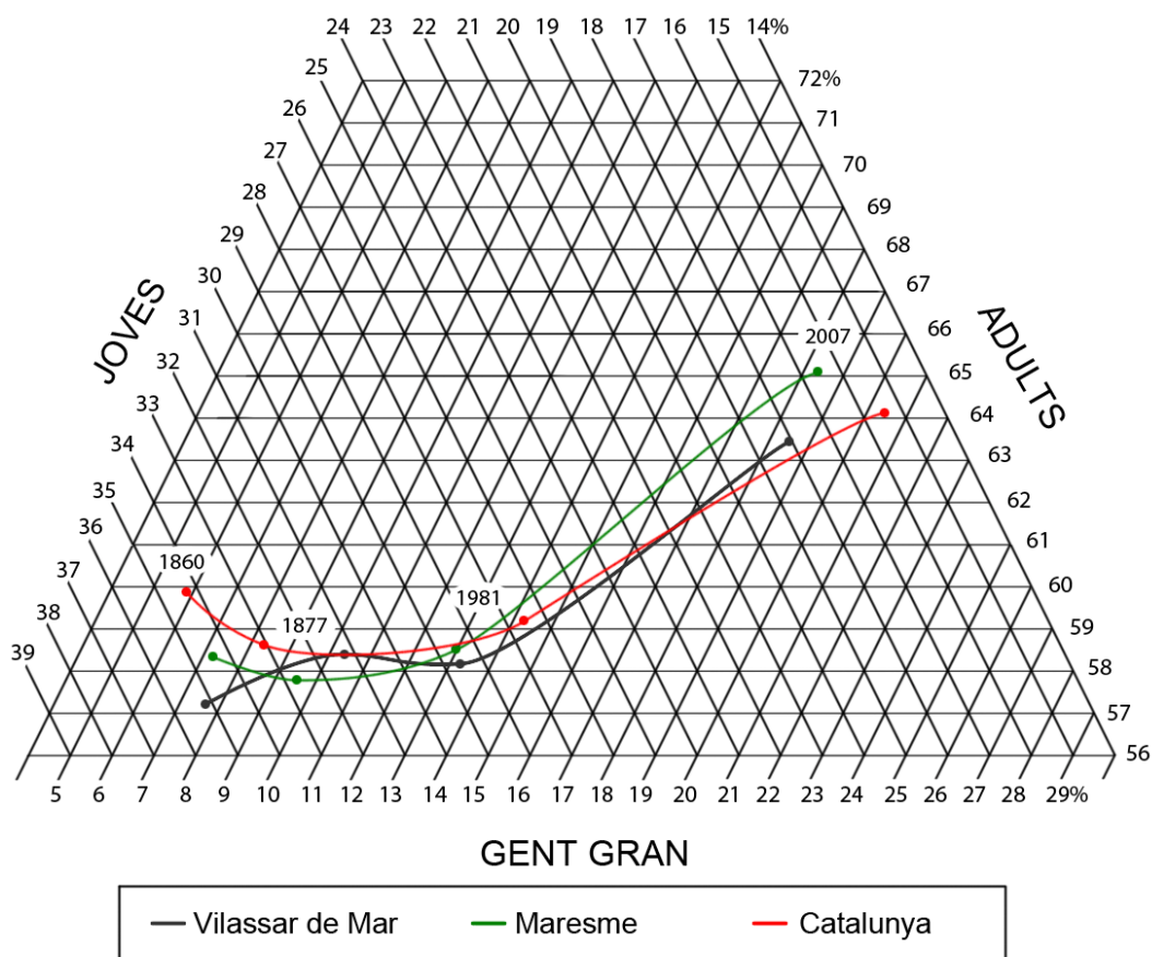
Diagrama 2.1.- Representació de l'evolució de la composició per edats de la població. Vilassar de Mar, Maresme i Catalunya, 1860, 1877, 1981 i 2007.
